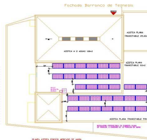
PLANTA AZOTEA EDIFICIO MERCADO DE HARIA
